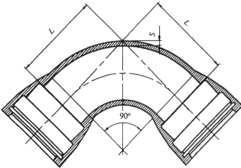
Рисунок Б.9 - Колено раструбное
