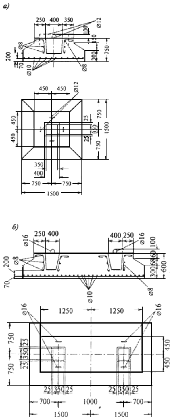
Рисунок 6.5 - Опорные железобетонные башмаки для труб диаметрами 400-500 мм под одну
