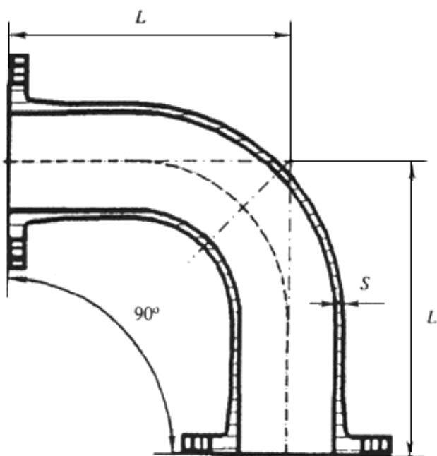
Рисунок Б.8 - Колено фланцевое
