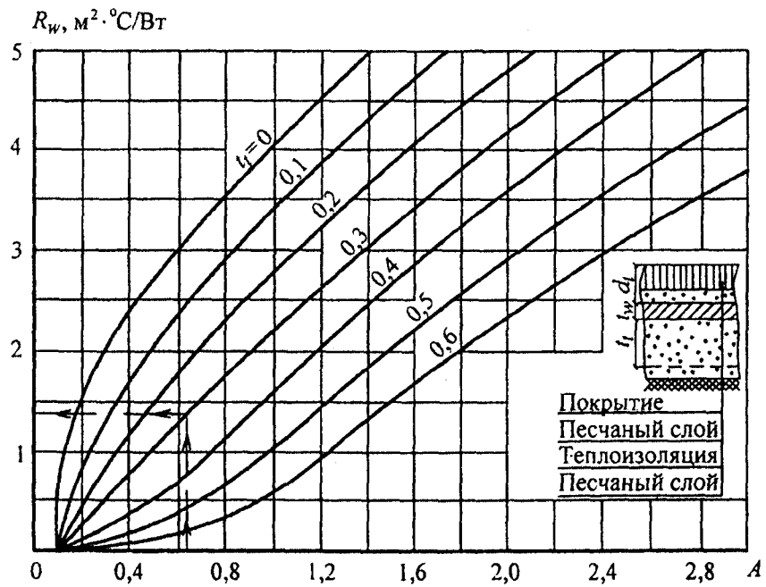
Рисунок Д.2 – Номограмма для определения термического сопротивления теплоизоляции
