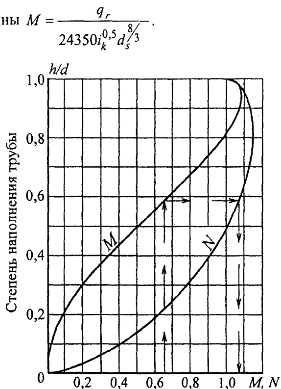
Рисунок Н.1 – График для определения коэффициента N и степени наполнения трубы (отношения глубины потока h к диаметру трубы d )
