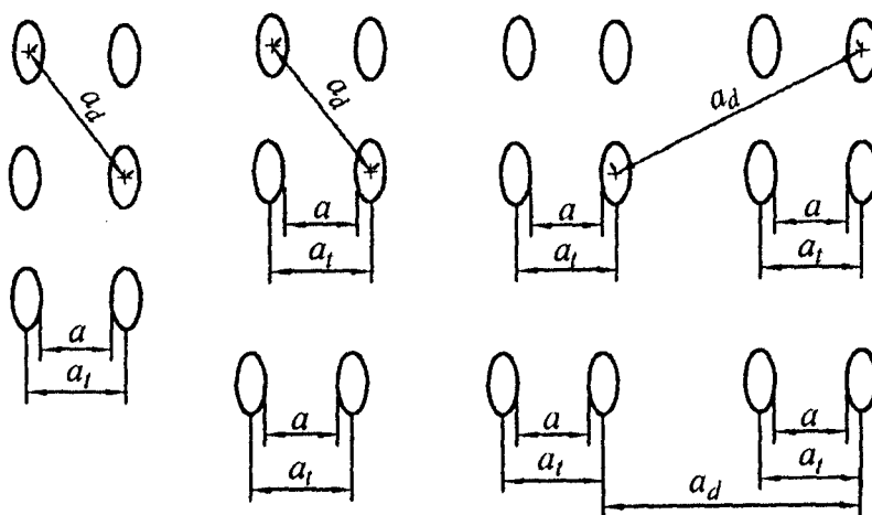
Рисунок К.7 – Расчетные расстояния a, a_1, a_d между колесами опор воздушных судов
