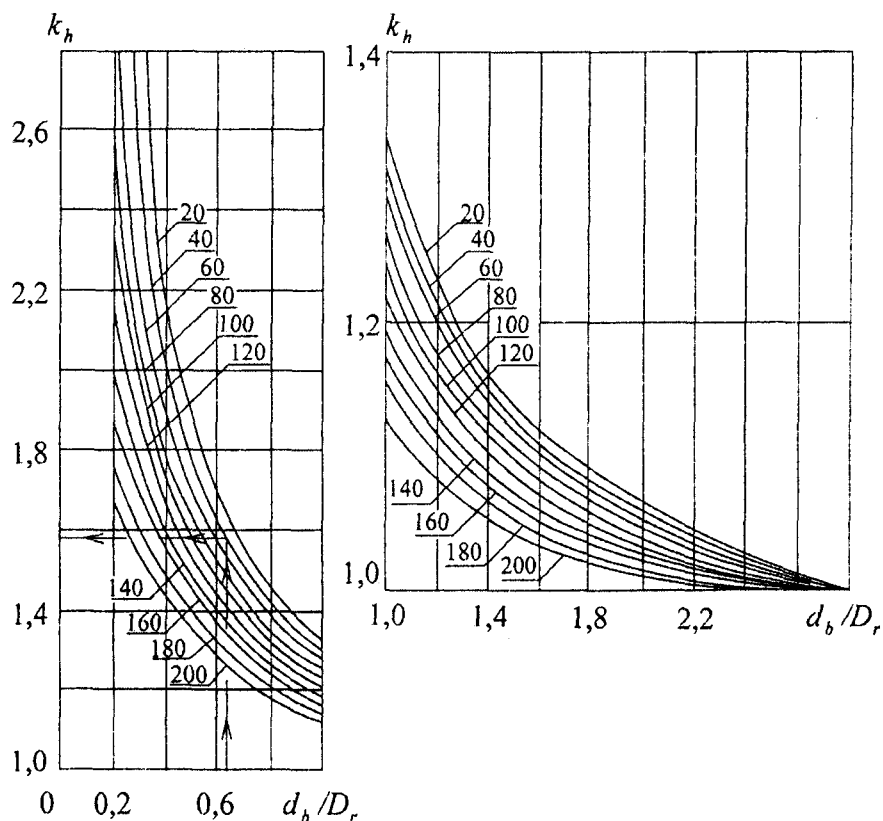
Рисунок Г.1 – График для определения коэффициента k_h жесткого массива. Цифрами на кривых указан коэффициент постели слоя основания K_{sr} , МН/м 3 , лежащего на жестком массиве
