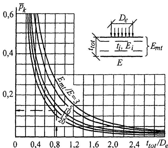
Рисунок Ж.1 – Номограмма для определения удельных контактных давлений \bar{p}_k на поверхности грунтового основания нежестких покрытий
