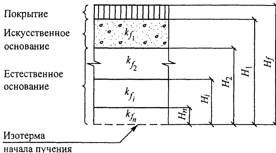
Рисунок Е.1 – Расчетная схема слоистого основания
