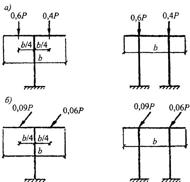
а - схема распределения вертикальной нагрузки; б - то же, горизонтальной нагрузки; P = pb - нормативная вертикальная нагрузка на опору или на соответствующий ярус опоры, где p - нормативное значение интенсивности вертикальной нагрузки на трассу, определяемое по формуле (52)
